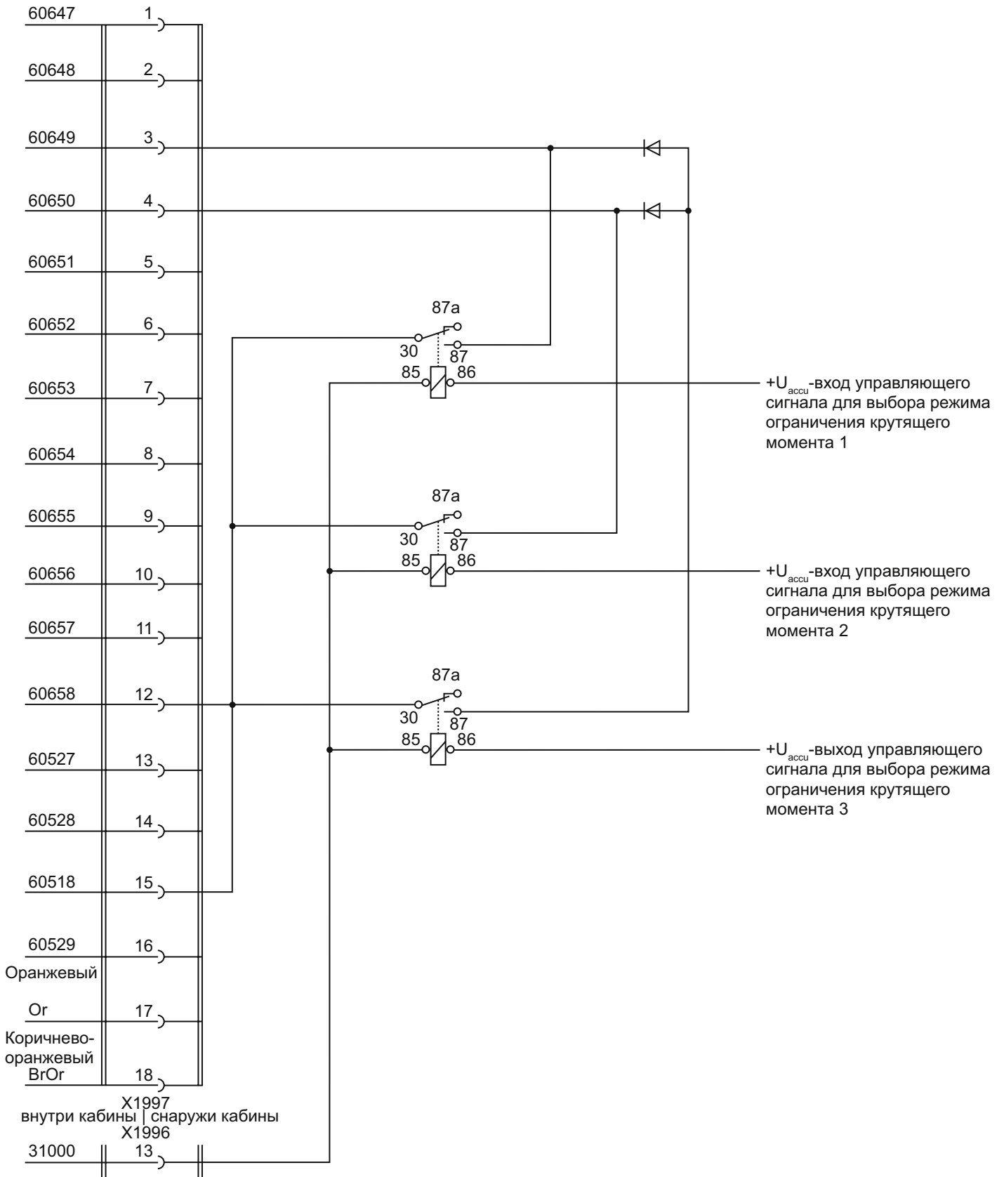
Пример схемы подключения для активирования режимов ограничения крутящего момента 1, 2 и 3
