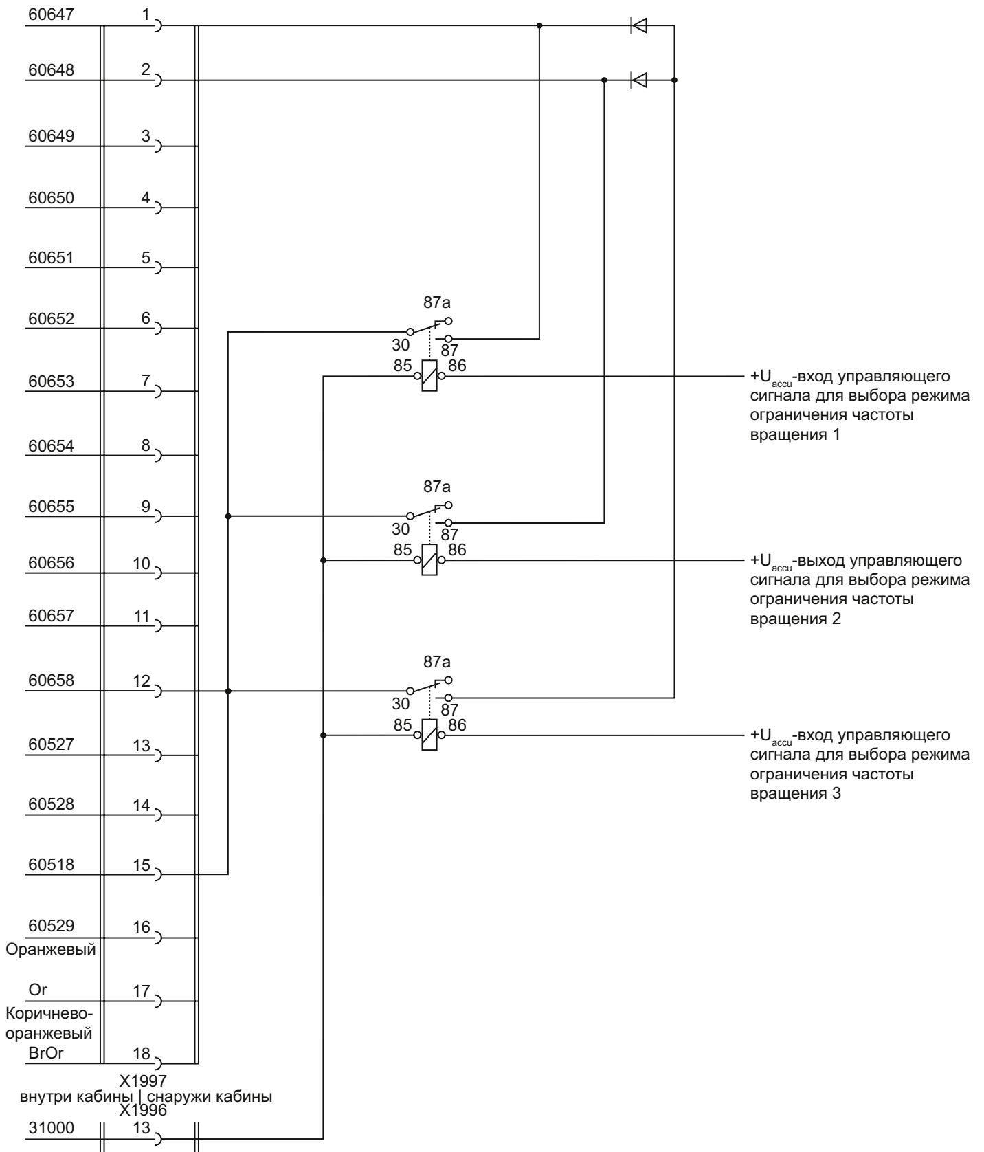
Пример схемы подключения для активирования режимов ограничения частоты вращения 1, 2 и 3
