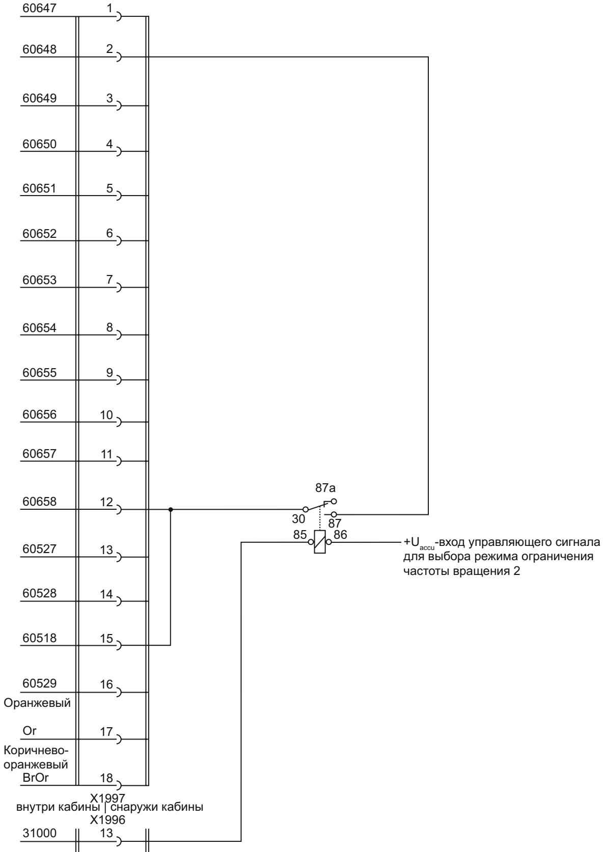
Пример схемы подключения для активирования режима ограничения частоты вращения 2
