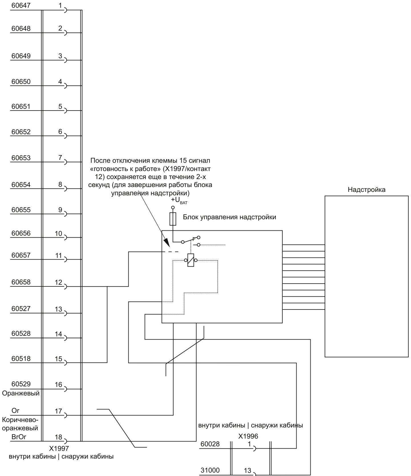
Пример схемы подключения электронного оборудования надстройки с помощью интерфейса CAN
