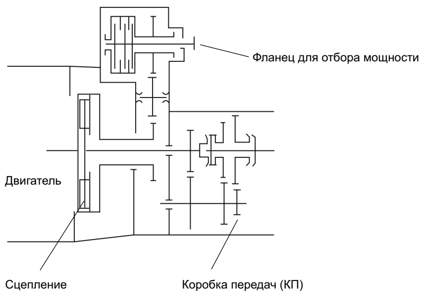
Рис 12: Схема подключения механизма отбора мощности NMV фирмы ZF ESC-072
