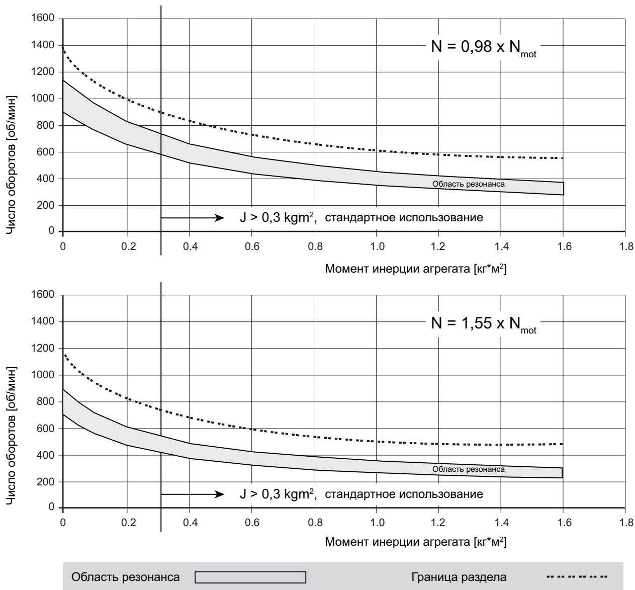
Рис 13: Механизм отбора мощности ZF NMV 221; зависимость резонансной частоты от момента инерции агрегата ESC-216_3 Работать в области резонанса нельзя ни при каких обстоятельствах!
