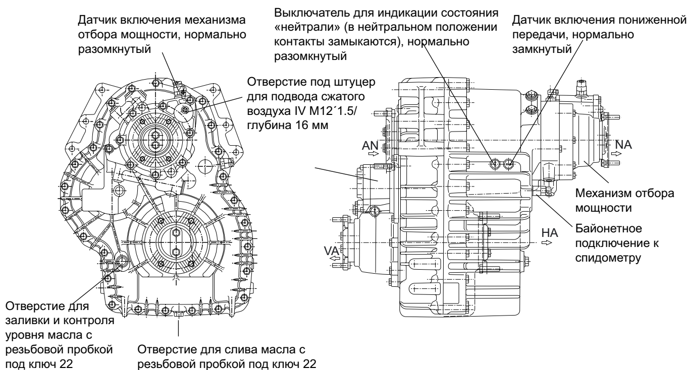
Рис 8: Отбор мощности от раздаточной коробки ESC-166
