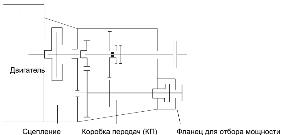
Рис 9: Пример: схема механизма отбора мощности зависимого от сцепления ESC-070
