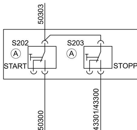
Рис 2: Подключение к «подготовке» для старта и остановки двигателя ESC-163
