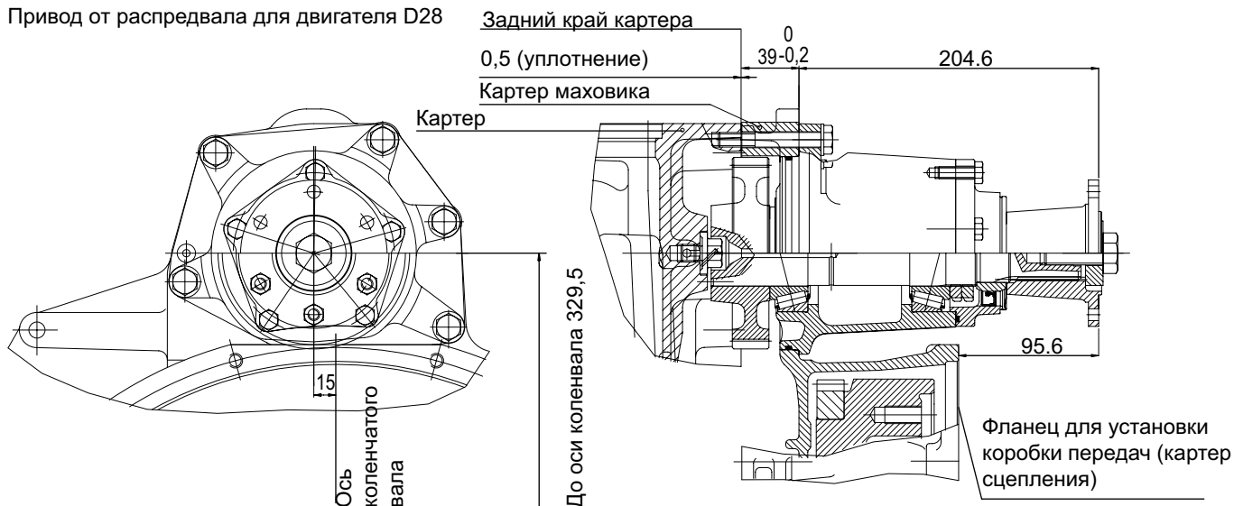
Рис 5: Привод от распредвала у двигателя D28 ESC-828
